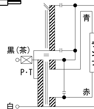
配線図
