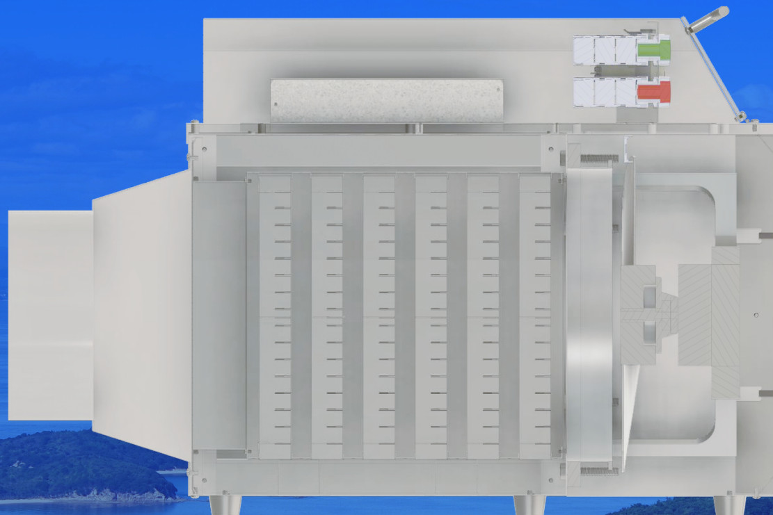
右側断面
